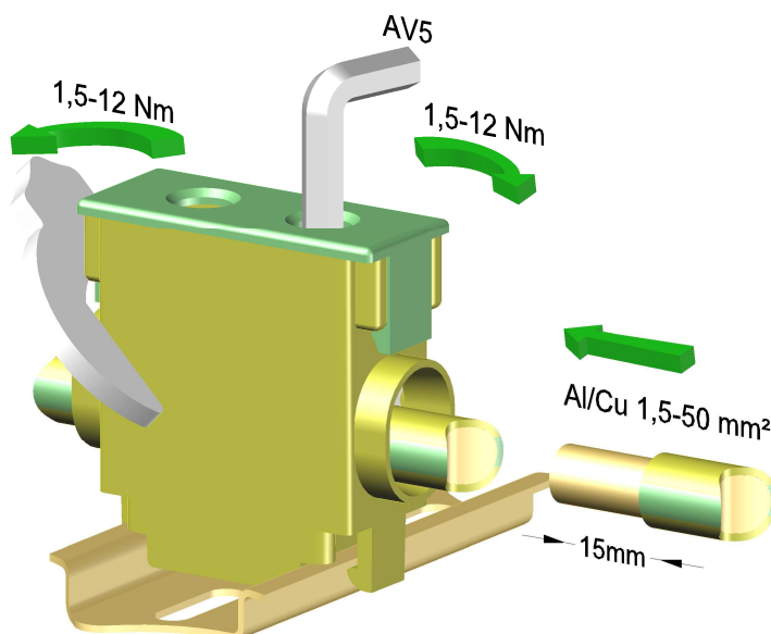
KIRISTYS- JA VASTAMOMENTTI TIGHTEN- AND REVERSE TORQUE
