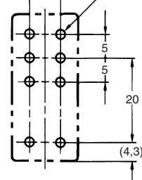
Otwory montażowe
