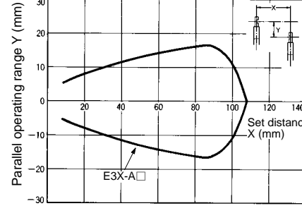
E32-T54
