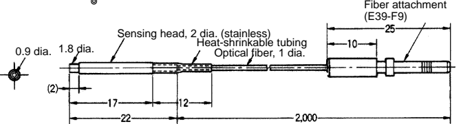
E32-T22L ✂
