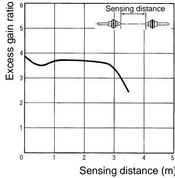
E32-T11L + E39-F2
