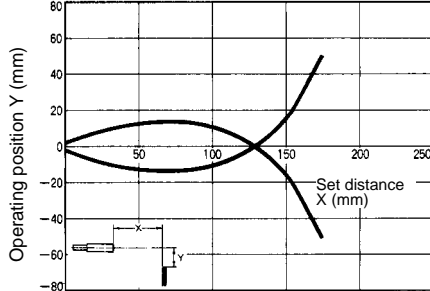
E32-D32L
