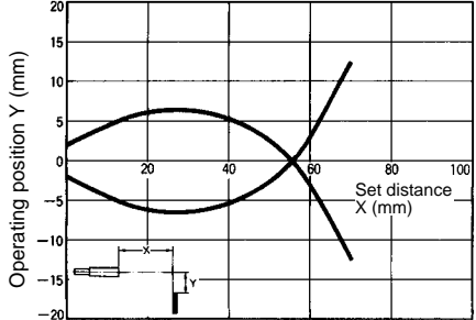
E32-D32
