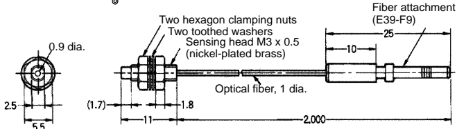
E32-TC200 ✂
