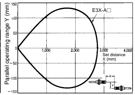
E32-T61 + E39-F1
