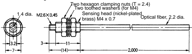
E32-T21L ✂
