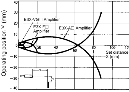
E32-D32L
