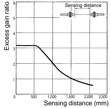
E32-T11L + E39-F3
