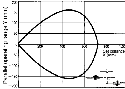
E32-T11
