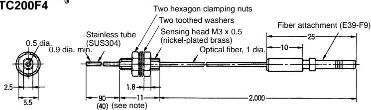
E32-TC200F ✂ E32-TC200F4
