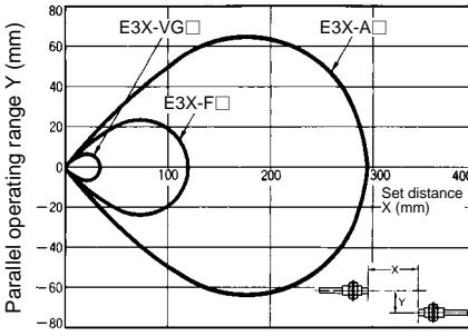
E32-T11
