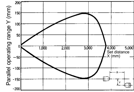
E32-T14
