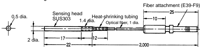
E32-T22 ✂
