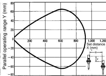
E32-TC200 + E39-F2
