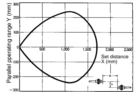
E32-T11L
