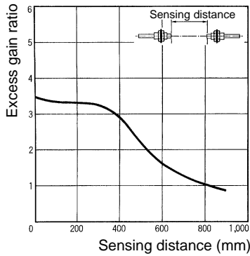
E32-T11L + E39-F1
