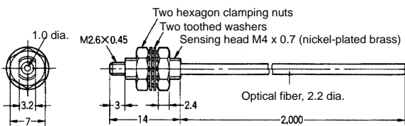
E32-TC200 ✂
