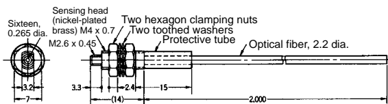
E32-T11 ✂
