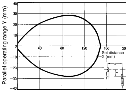
E32-T24
