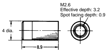
E39-F1 Long-distance Lens Unit
