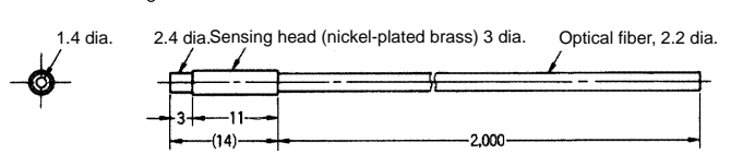
E32-T12L ✂
