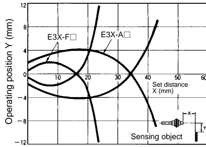
E32-D73
