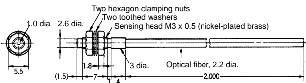
E32-TC200A ✂
