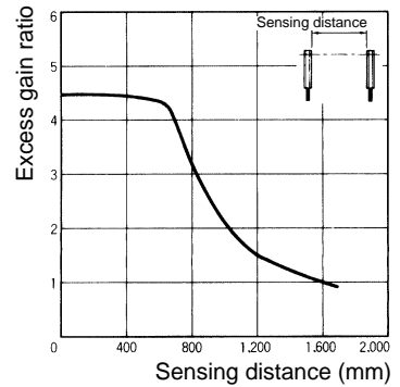
E32-T24S
