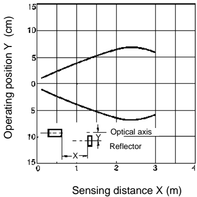
E3JK-R2□□
