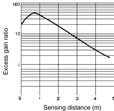
E3JK-R4□□
