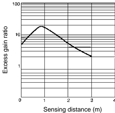
E3JK-R2□□
