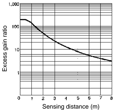
E3JK-5□□
