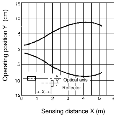
E3JK-R4□□
