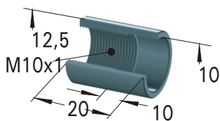
tulejka zderzaka
