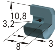
głowica łącząca
