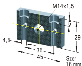
kołnierz uniwersalny
