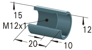
tulejka zderzaka
