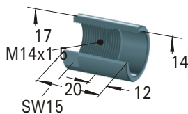
tulejka zderzaka
