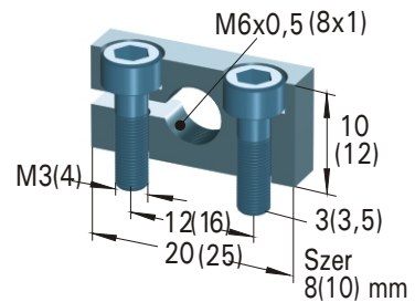
kołnierz zaciskowy
