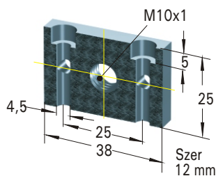
kołnierz uniwersalny
