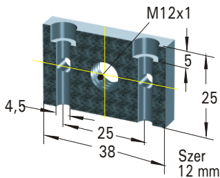
kołnierz uniwersalny
