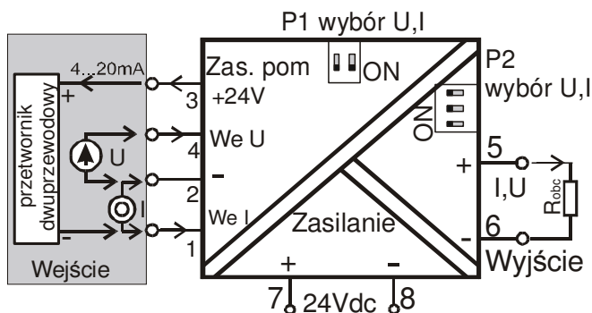
Opis zacisków podłączeniowych
