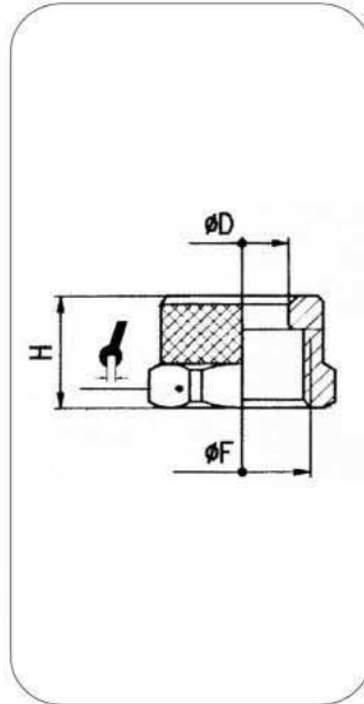
ART. 310 Dado di serraggio Locking nut
