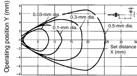
E32-D22L with E3X-NM11
