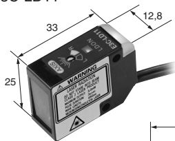
E3C-LD11
