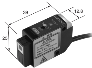
E3C-LR11
